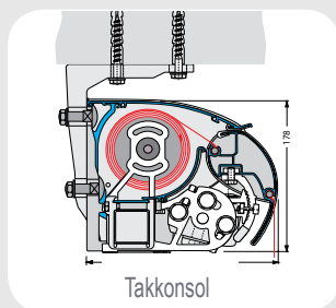
Väggkonsol
