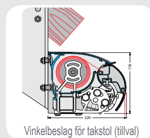
Takkonsol
